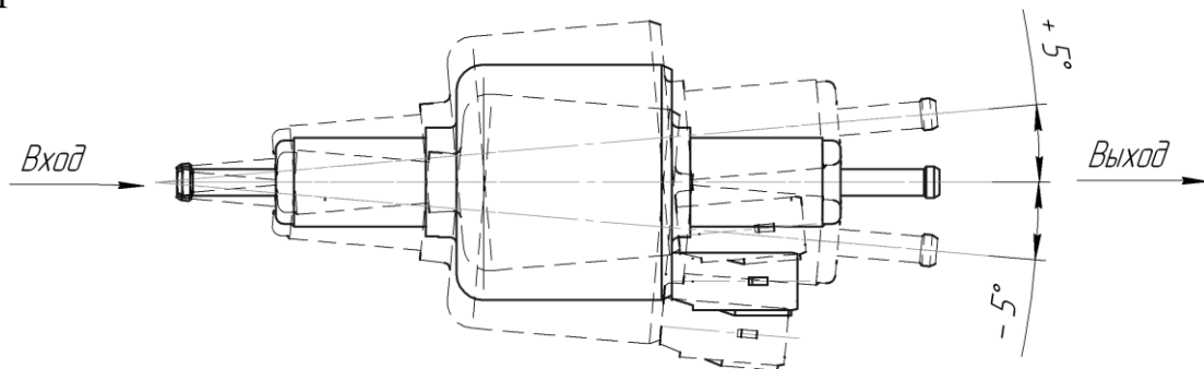
Рис. 8.4а Допустимое монтажное положение топливного насоса
