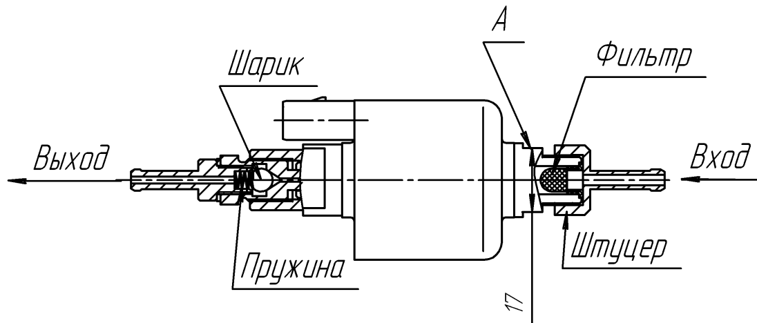
Рис.10 – Топливный насос
