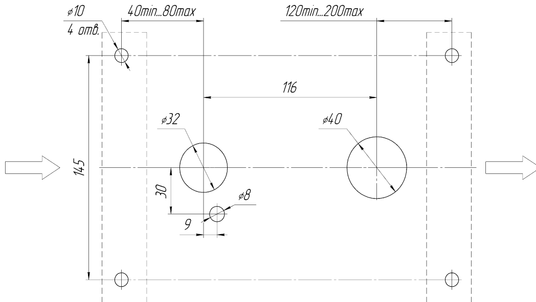
Рис. 8.1б – Монтажные отверстия для установки нагревателя
